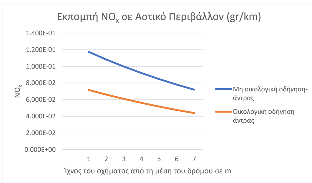
Διάγραμμα 5.6α: Επιρροή ίχνους του οχήματος από τη μέση της οδού σε αστικό δίκτυο, με οικολογική και μη οικολογική συμπεριφορά οδήγησης, όταν ο οδηγός είναι άντρας (AvgTTC=15)
