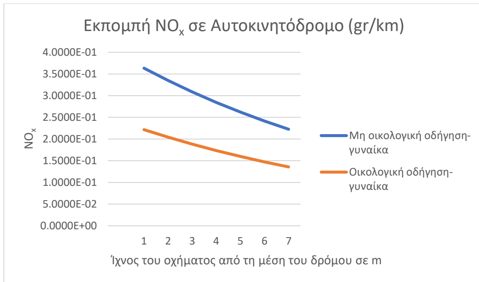
Διάγραμμα 5.5β: Επιρροή ίχνους του οχήματος από τη μέση της οδού σε αυτοκινητόδρομο, με οικολογική και μη οικολογική συμπεριφορά οδήγησης, όταν ο οδηγός είναι γυναίκα (AvgTTC=15)
